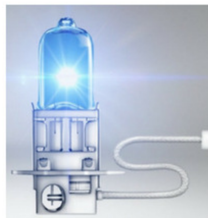
O64151CBI LAMPARA H3 CBI 12v 55W PK22S
